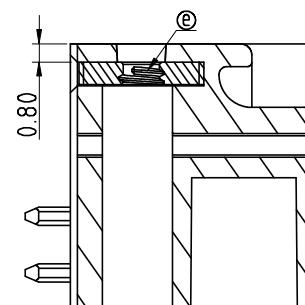
SECTION 0-0
