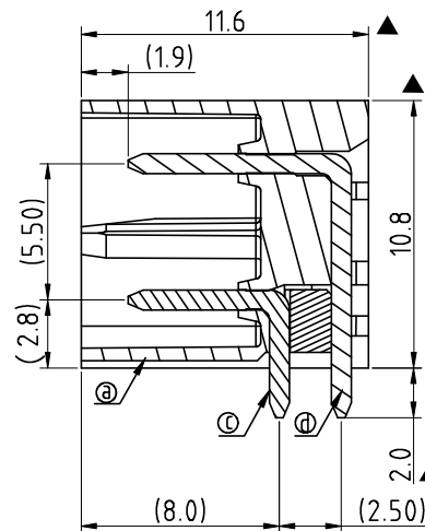
SECTION 0-0
