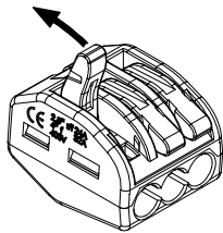
Step 1. 打开压板 Open the lever
