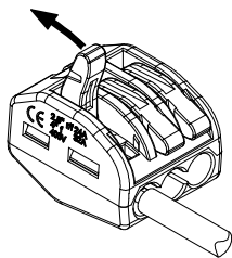
Step 1. 打开压板 Open the lever
